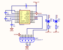
UART
